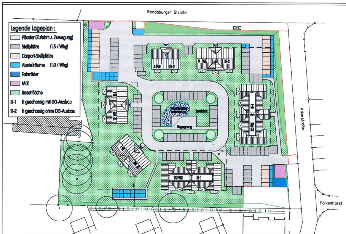
Abbildung 5: Vorentwurf Lageplan 05.04.2018: Quelle: Arch.- u. Ing. Büro Bernd Löhmann, Bad Segeberg
